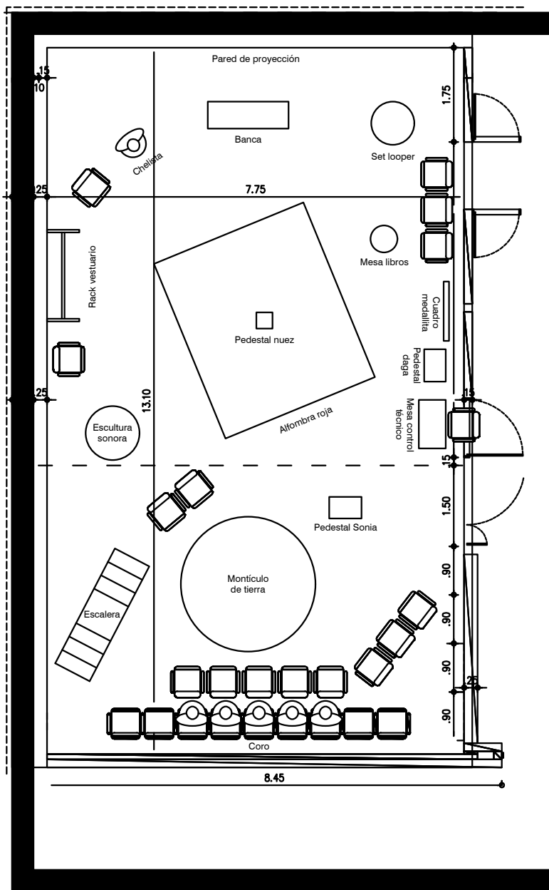
Plano Escenográfico Luna MAPET - Esc: 1:100
